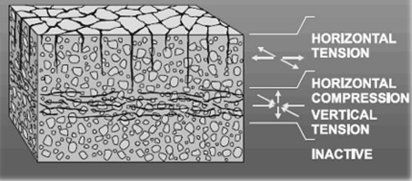
Agrietamiento diseminado (mapeo)
