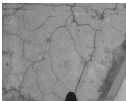
(a) fissuras primárias no piso da tomada d'água da UHE Paulo Afonso III
